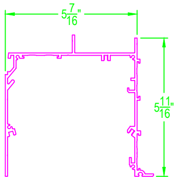
POCKET - AXP355L
