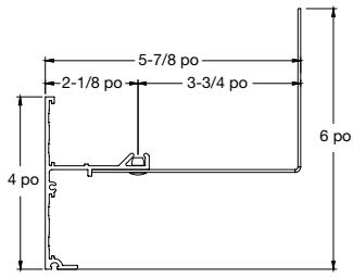
Plafond à plafond Classique
