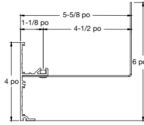
Plafond au mur Classique
