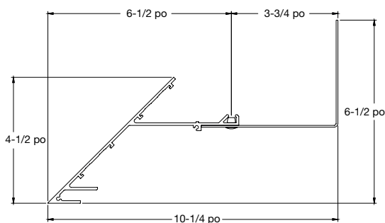
Plafond à plafond Knife Edge MD Tranchant
