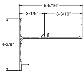
Installation de panneaux Vector MD Plafond à plafond Classique 4 po
