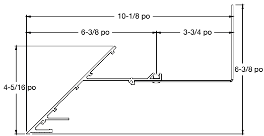
Plafond à plafond Knife Edge MD Tranchant pour gypse
