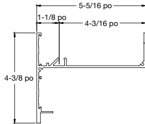
Installation de panneaux Vector plafond au mur Classique 4 po
