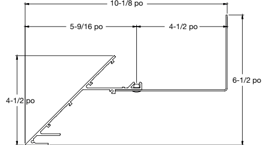
Plafond au mur Knife Edge MD Tranchant
