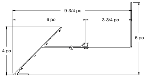
Plafond à plafond Knife Edge MD Tranchant
