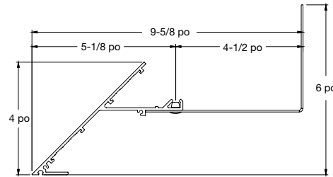
Plafond au mur Knife Edge MD Tranchant
