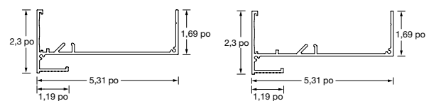
Classique plafond-mur
