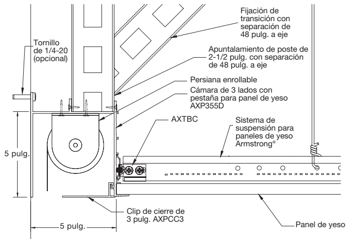
Cámara para persianas/cortinas manuales – Para sujeción con postes de 2-1/2"
