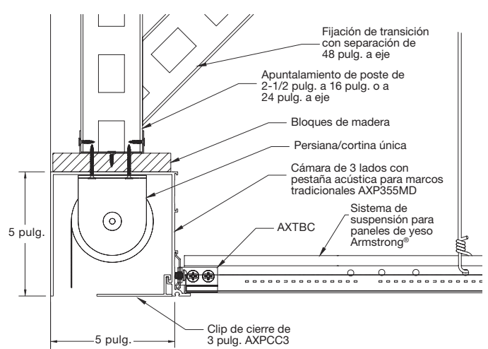
Cámara para persianas/cortinas manuales – Para marcos tradicionales
