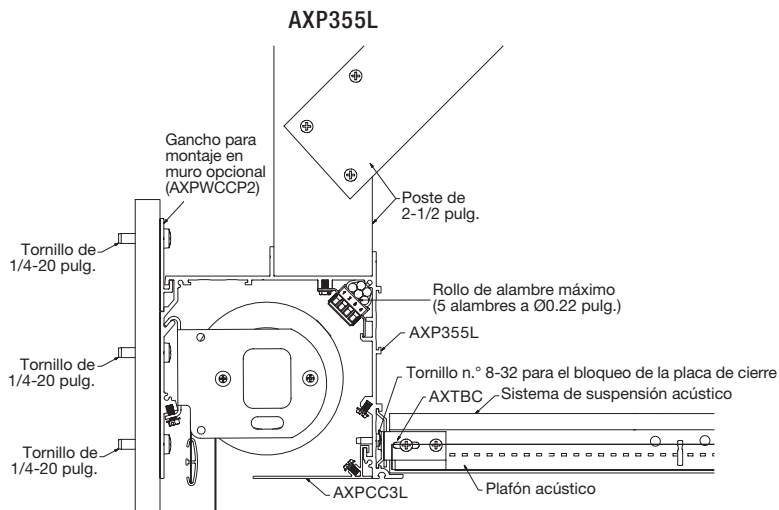
Cámara para persianas/cortinas motorizadas – Para sujeción con postes de 2-1/2"
