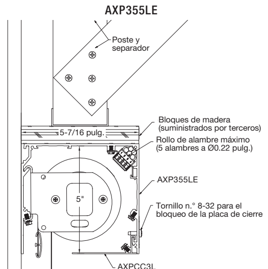
Cámara para persianas/cortinas motorizadas – Para marcos tradicionales
