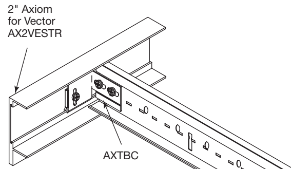
AXTBC – T-Bar Connector Clip
