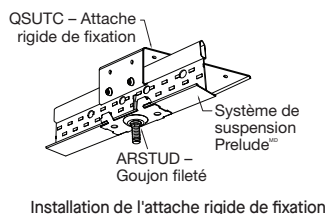
Installation de l'attache rigide de fixation
