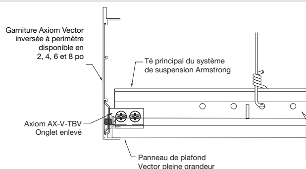
② Panneau complet Vector avec garniture de périmètre inversée Axiom Vector
