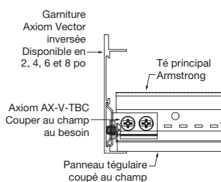
④ Panneau coupé téguilaire avec garniture de périmètre inversée Axiom Vector
