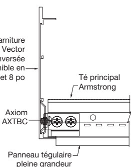
⑤ Panneau complet téguilaire avec garniture de périmètre inversée Axiom Vector
