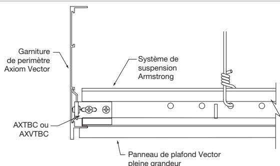
① Panneau complet de plafond Vector avec garniture de périmètre Axiom Vector
