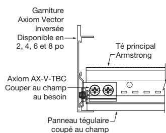
③ Panneau coupé Vector avec garniture de périmètre inversée Axiom
