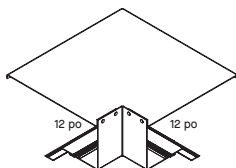
Tranchant Knife Edge d'un plafond au mur Coin intérieur
