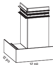
Classique d'un plafond à plafond Coin extérieur
