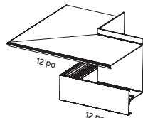
Classique d'un plafond au mur Coin intérieur
