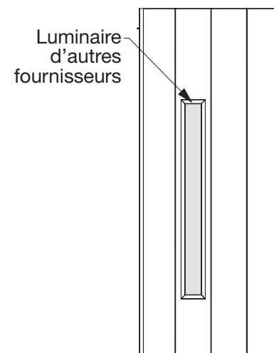
Option 2 L'éclairage est encastré dans le panneau.
