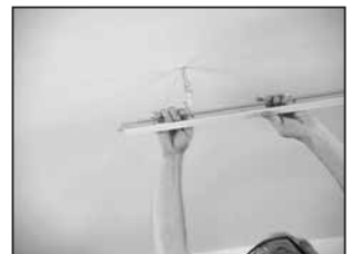
Installer le premier longeron principal
