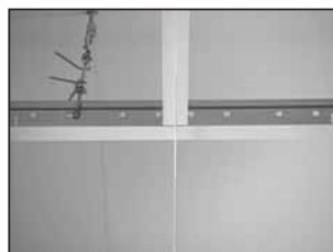
Aligner la deuxième ficelle de guidage avec le premier té croisé de quatre pieds
