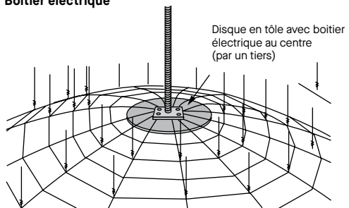
Boîtier électrique
