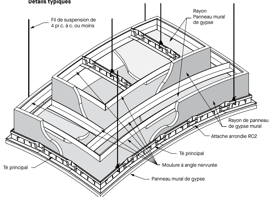
Détails typiques
