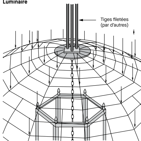
Luminaire
