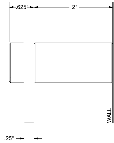
Dimensiones del Panel para Paredes y de los Componentes
