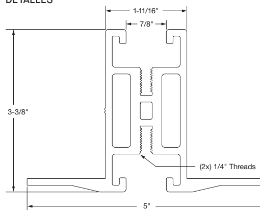
Perfil de Skylo Plenum Cap de 5"
