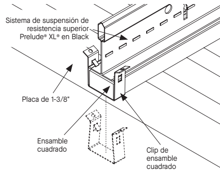
Ensamblaje de Ensamble Cuadrado de plafón
