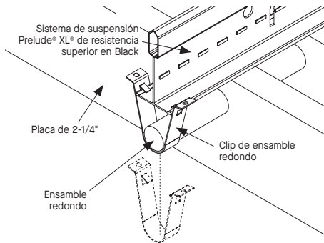
Ensamblaje de Ensamble Redondo de plafón
