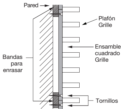
Ensamblaje de Ensamble cuadrado para pared
