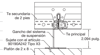
Detalle de instalación: sistema de plafón oculto
