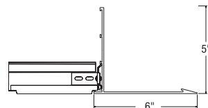
Perfil Axiom Knife Edge (AXKE5STR)
