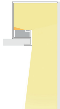
Cornisa para pared
