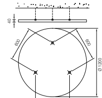
Circle Ø 1200 x 40 mm
